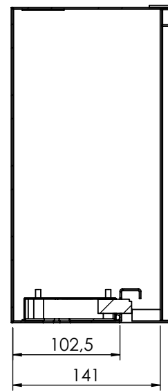
PRZEKRÓJ A-A
