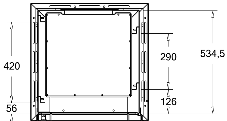
Przekrój F-F
