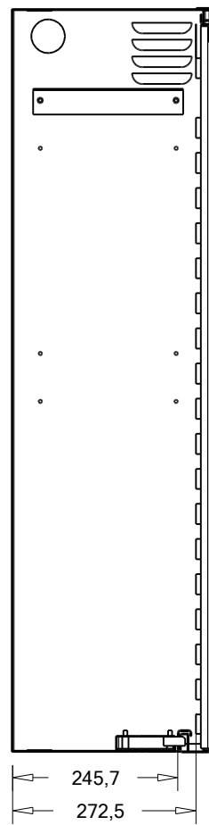
Przekrój J-J
