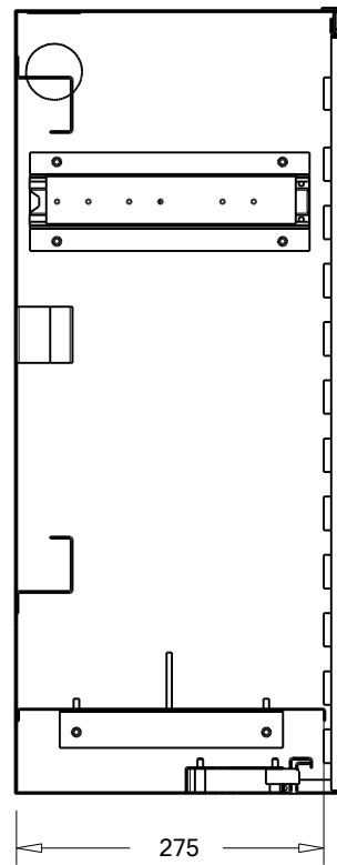
Przekrój B-B
